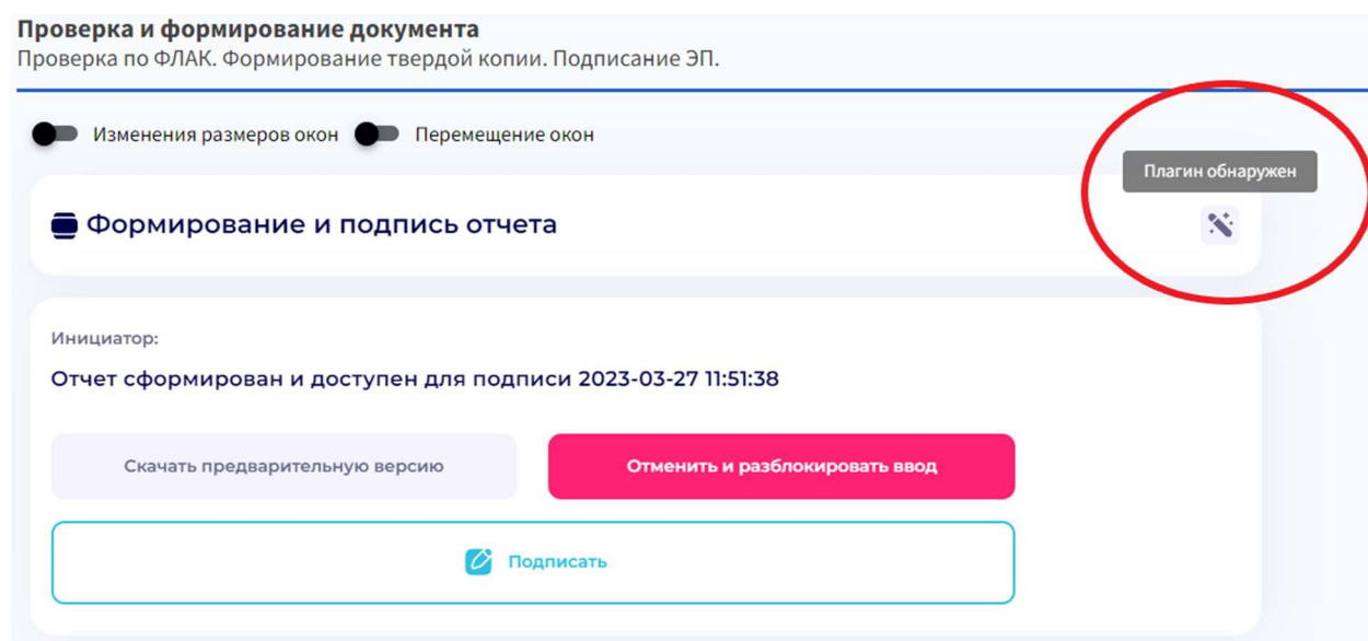
Рисунок 37 Плагин обнаружен
