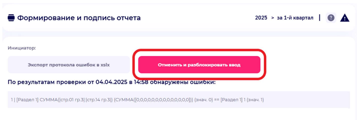
Рисунок 31 Отмена блокировки
