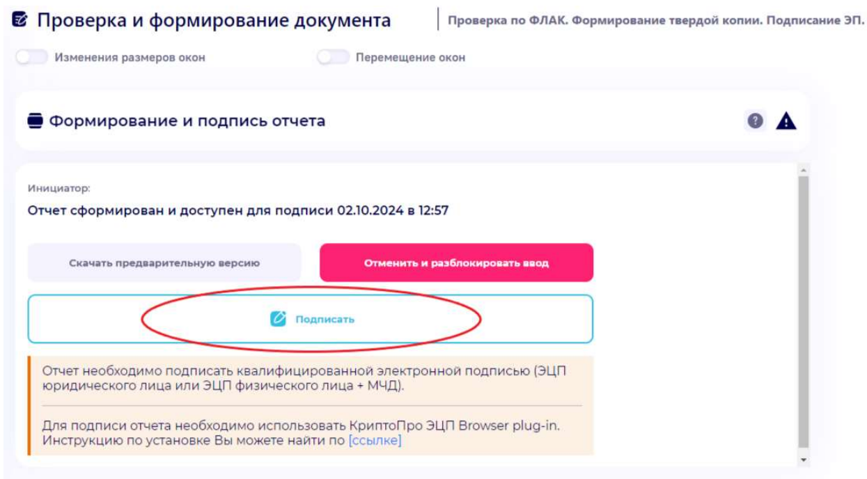
Рисунок 38 Кнопка "Подписать"
