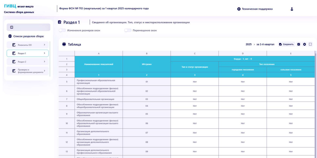
Рисунок 8 Заполнение раздела
