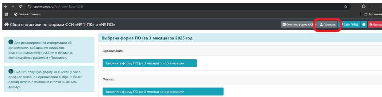
Рисунок 5 Кнопка "Профиль"
