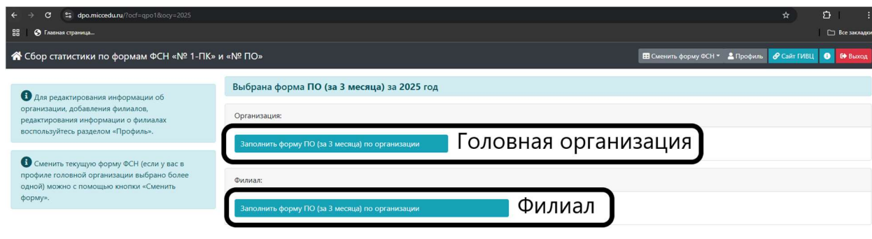
Рисунок 10 Заполнение формы
