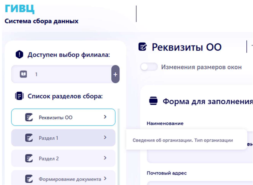
Рисунок 7 Наименование раздела
